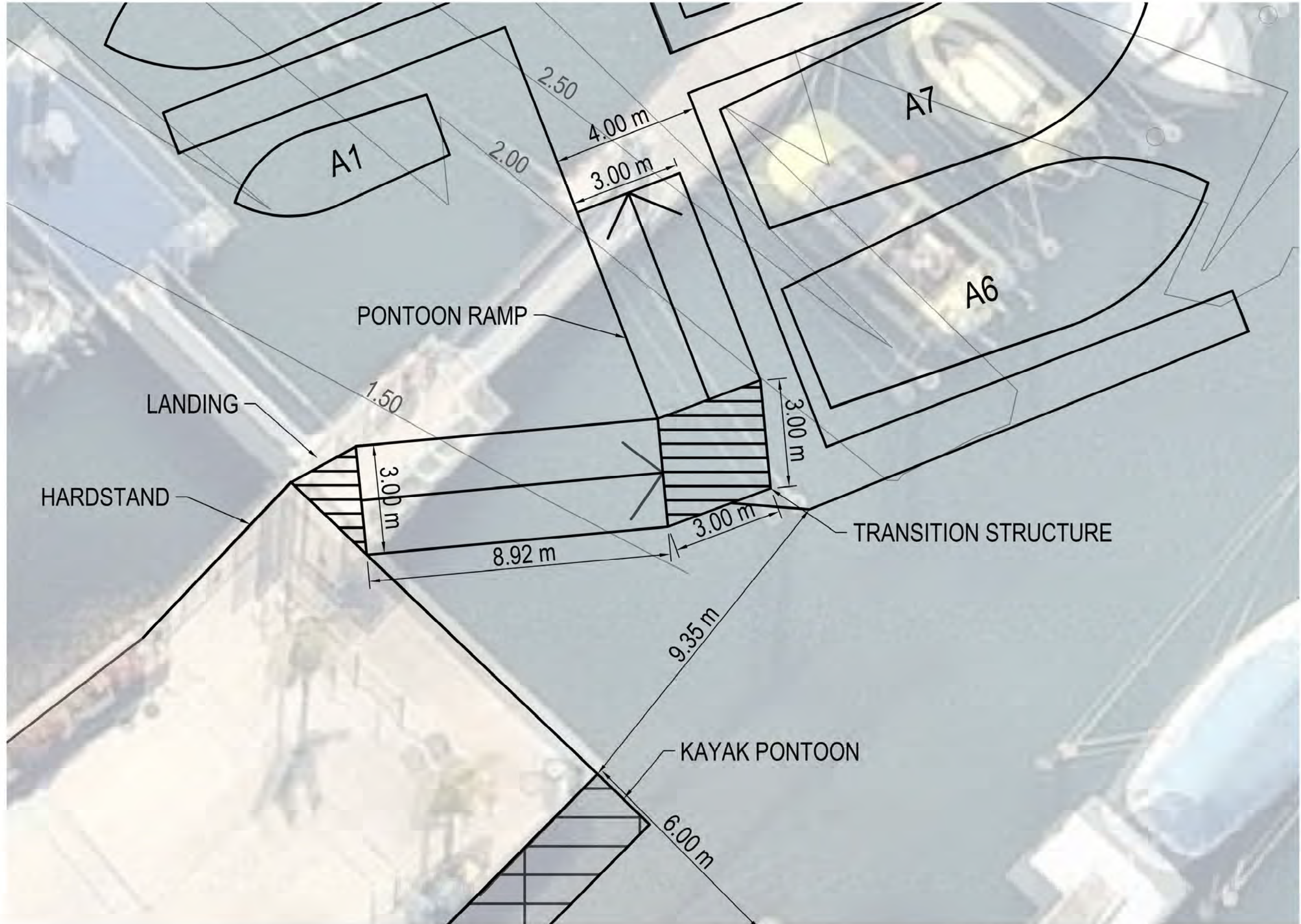
GANGWAY LAYOUT SCALE 1:100
